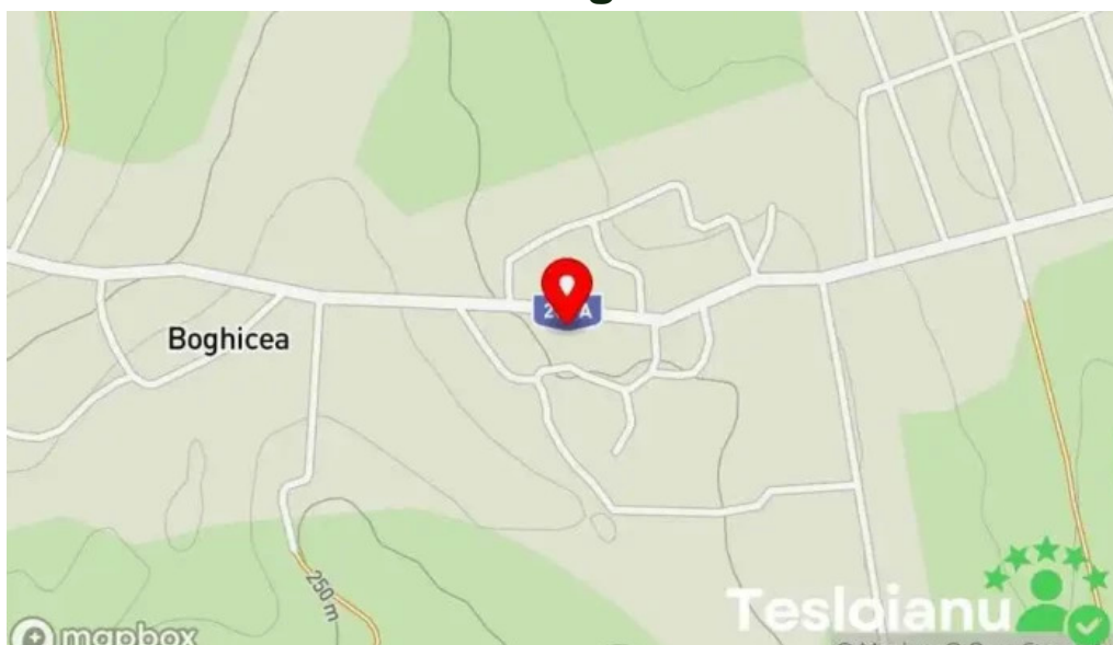
Boghicea hart?
