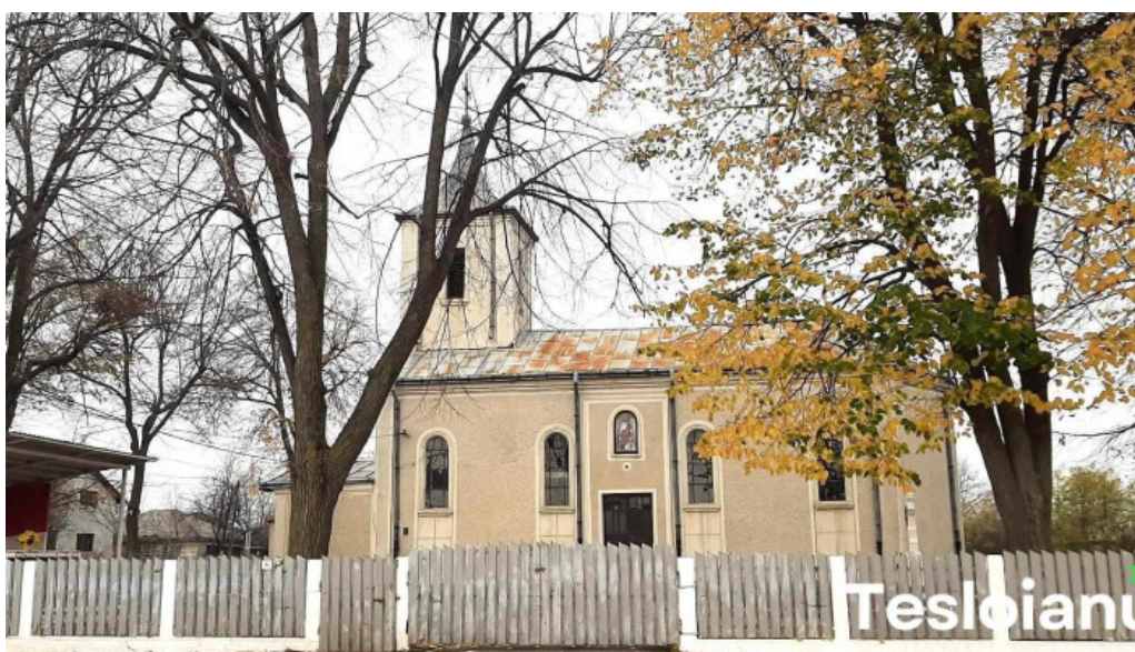
Boghicea boghicea
