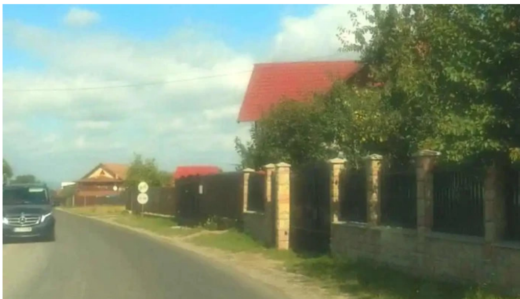
Carpinis videoclipuri
