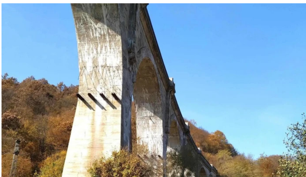
Viaductul luncoiu de jos aproape de mine
